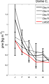
prw_DC_CM6015-LR-amip-split-G-02_1999_2008
