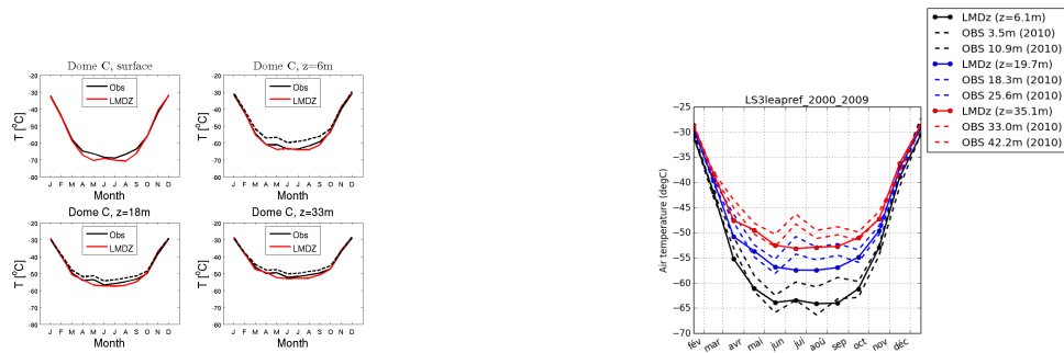
temp_DC_LS3leapref_2000_2009
