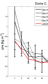
prw_DC_LS3leapref_2000_2009
