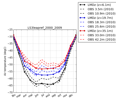
tempDC-LS3leapref_2000_2009
