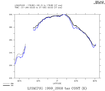
LS3MIPJG_1999_2008_con
