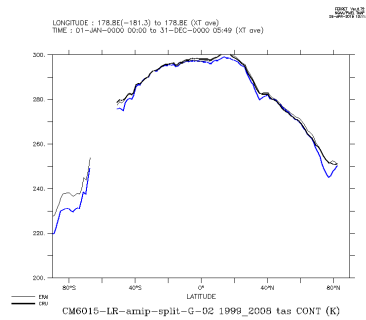
CM6015-LR-amip-split-G-02_1999_2008_con
