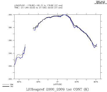
LS3leapref_2000_2009_con
