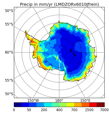
precipSH-LMDZORv6010Jfrein
