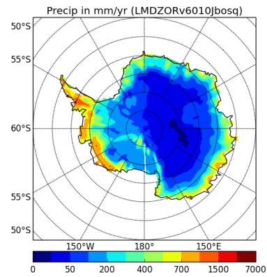
precipSH-LMDZORv6010Jbosq
