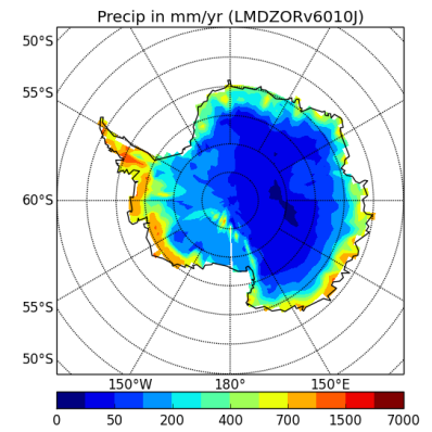
precipSH-LMDZORv6010J
