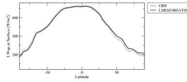
rluszon
