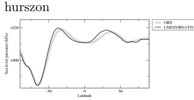
pslzon
