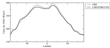
rlutscszon
