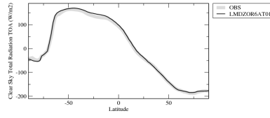
rttczon
