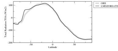
rttzn
