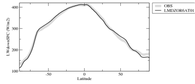
rldszon
