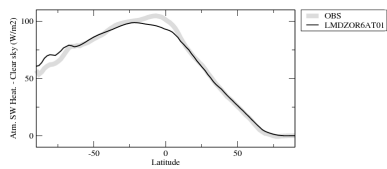
rsahcszon
