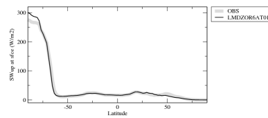
rsuszon
