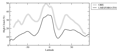
chlcalipsozon
