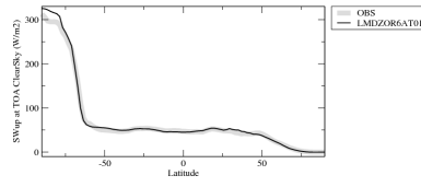
rsutczon
