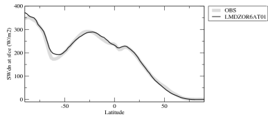
rsdszon
