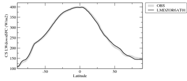
rldscszon
