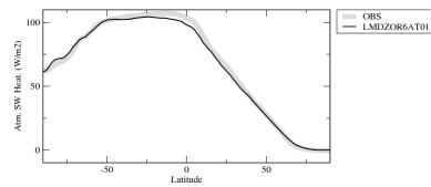
rsahzon
