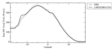
rsttzn
