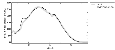
rstszon
