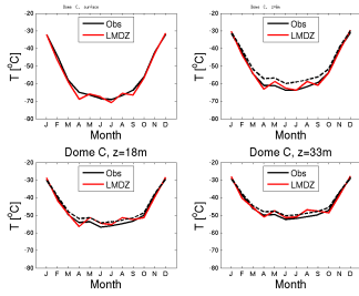
temp_DC_LMDZOR6AT01_1980_1980
