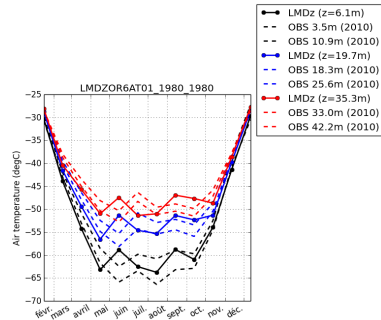
tempDC-LMDZOR6AT01_1980_1980
