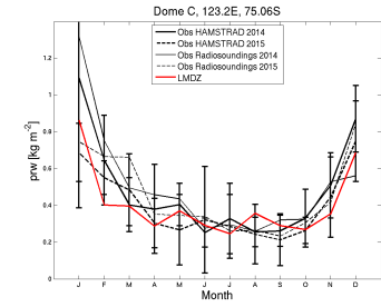
LWdnSFC_DC_LMDZOR6AT01_1980_1980 prw
