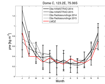
LWdnSFC_DC_LMDZOR6AT00_1980_1980 prw
