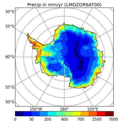
precipSH-LMDZOR6AT00
