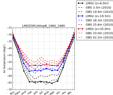
tempDC-LMDZOR14ttopB_1980.1989
