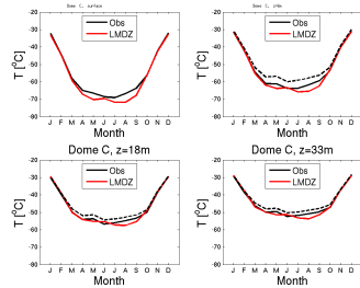
temp_DC_LMDZOR14splith_1980.1989
