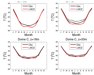
temp_DC_LMDZOR14splithB_1980.1989
