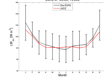
LWdnSFC_DC_LMDZOR14httop_1980.1989
