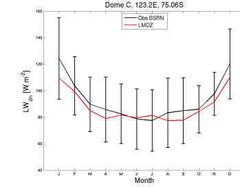
LWdnSFC_DC_LMDZOR14ttopB_1980.1989
