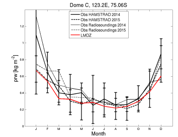
prw_DC_LMDZOR14splith_1980.1989
