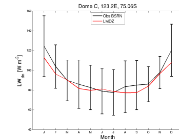
LWdnSFC_DC_LMDZOR14splithB_1980.1989
