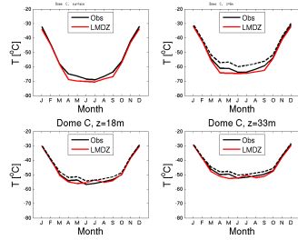
temp_DC_LMDZOR14httop_1980.1989
