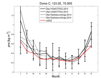
prw_DC_LMDZOR14splithB_1980.1989
