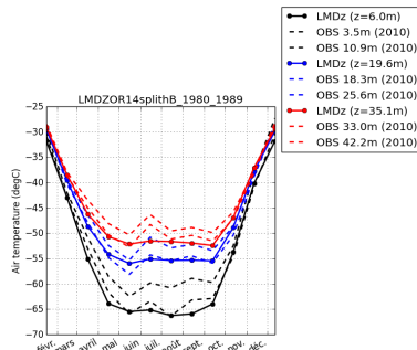
tempDC-LMDZOR14splithB_1980.1989
