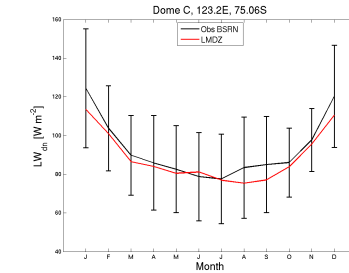
LWdnSFC_DC_LMDZOR14splith_1980.1989
