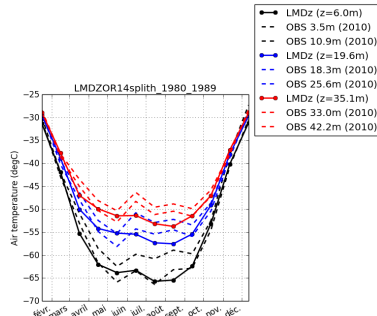
tempDC-LMDZOR14splith_1980.1989
