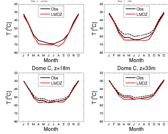
temp_DC_LMDZOR14ttopB_1980.1989
