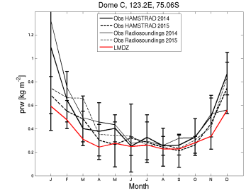
prw_DC_LMDZOR14ttopB_1980.1989
