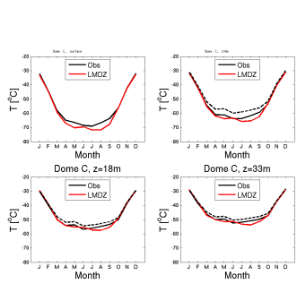
temp_DC_LMDZOR14splith_1980-1989
