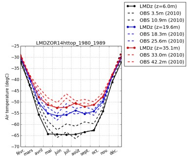
tempDC-LMDZOR14http_1980-1989
