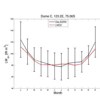
LWdnSFC_DC_LMDZOR14http_1980-1989
