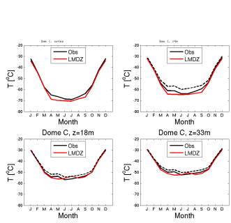
temp_DC_LMDZOR14http_1980-1989
