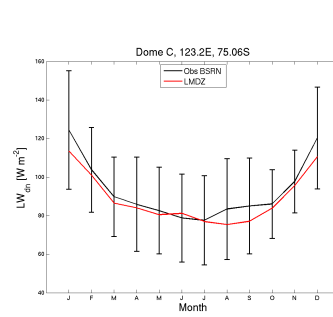
LWdnSFC_DC_LMDZOR14splith_1980-1989
