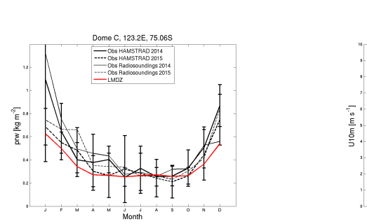
prw_DC_LMDZOR14http_1980-1989
