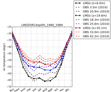
tempDC-LMDZOR14splith_1980-1989
