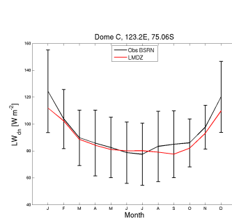
LWdnSFC_DC_LMDZOR14splitD_1980-1989
