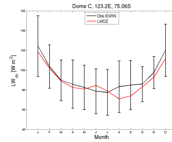
LWdnSFC_DC_LMDZORv6011cvoroH.1980.1984
