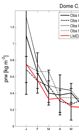
prw_DC_LMDZ
