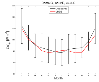
LWdnSFC_DC_LMDZORv6011gustH.1980.1984
