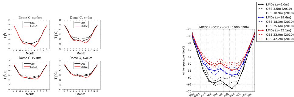
temp_DC_LMDZORv6011cvoroH.1980.1984
