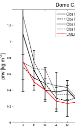
prw_DC_LMDZORv6011gustH.1980.1984
