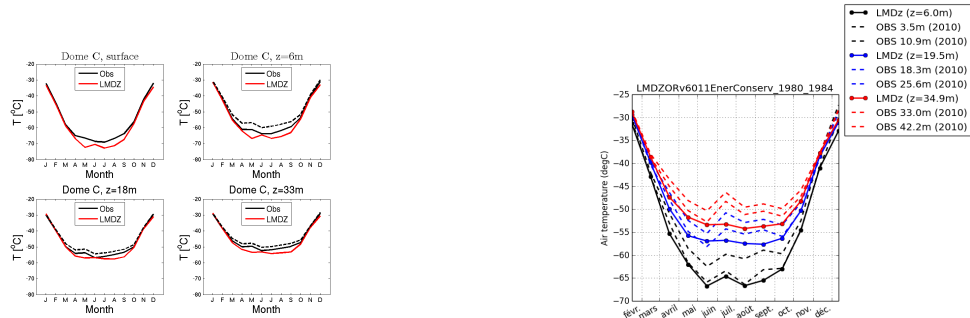
temp_DC_LMDZORv6011EnerConserv_1980_1984
