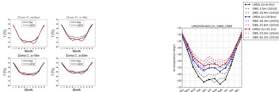
temp_DC_LMDZORv6011H.1980.1984
