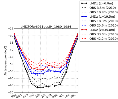
tempDC-LMDZORv6011gustH.1980.1984
