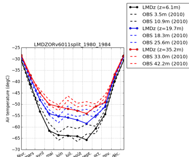
tempDC-LMDZORv6011split_1980_1984
