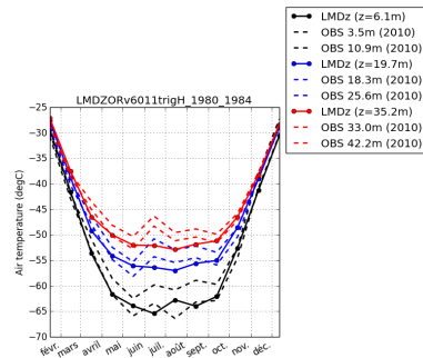
tempDC-LMDZORv6011trigH.1980.1984
