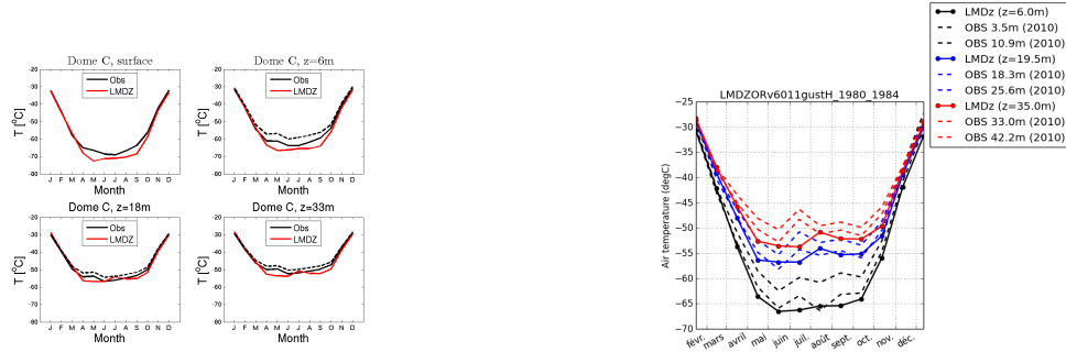
temp_DC_LMDZORv6011gustH.1980.1984
