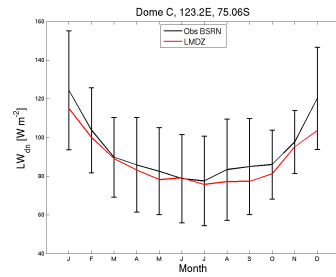
LWdnSFC_DC_LMDZORv6011EnerConserv_1980_1984
