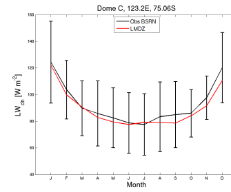
LWdnSFC_DC_LMDZORv6011trigH.1980.1984
