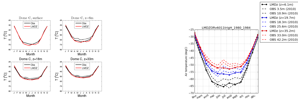
temp_DC_LMDZORv6011trigH.1980.1984
