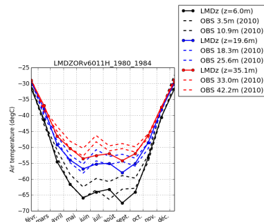
tempDC-LMDZORv6011H.1980.1984
