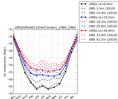
tempDC-LMDZORv6011EnerConserv_1980_1984
