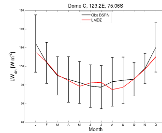
LWdnSFC_DC_LMDZORv6011H.1980.1984
