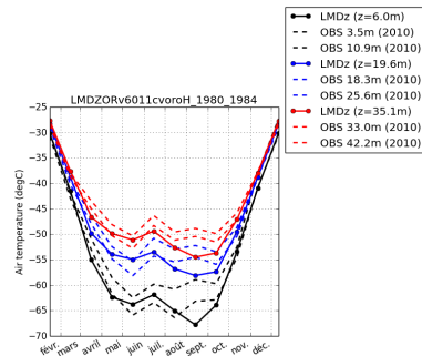
tempDC-LMDZORv6011cvoroH.1980.1984
