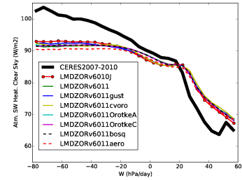
rsahcs_LMDZOR6011
