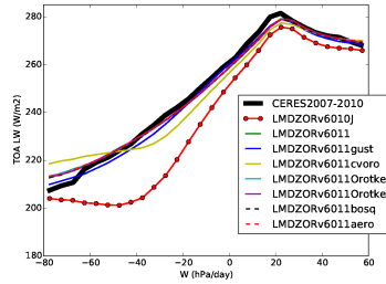
rlut_LMDZOR6011
