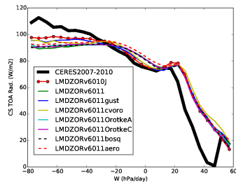
rttcs_LMDZOR6011
