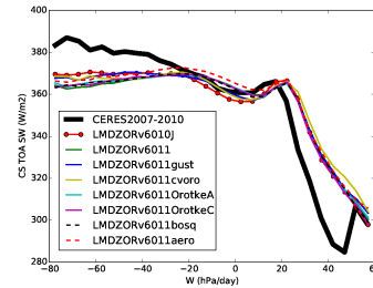
rsttcs_LMDZOR6011
