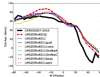
rtt_LMDZOR6011
