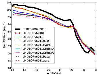
rsah_LMDZOR6011
