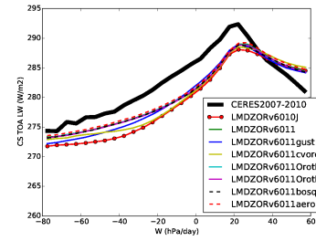
rlutcs_LMDZOR6011
