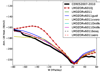
rlah_LMDZOR6011
