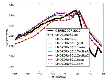
rstt_LMDZOR6011
