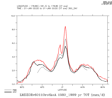
LMDZORv6011OrotkeA.1980_1999_tot
