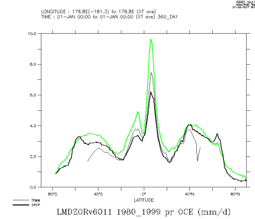
LMDZORv6011_1980_1999_oce
