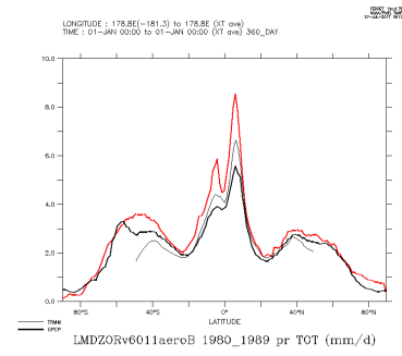
LMDZORv6011aeroB.1980_1989_tot
