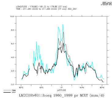
LMDZORv6011bosq.1980_1999_mix
