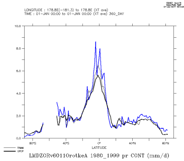
LMDZORv6011OrotkeA.1980_1999_con
