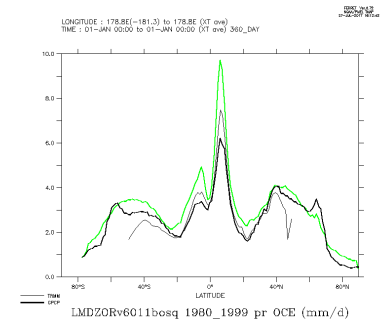
LMDZORv6011bosq.1980_1999_oce
