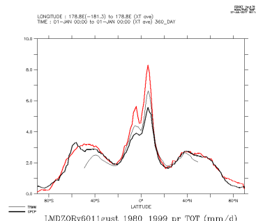
LMDZORv6011gust_1980_1999_tot
