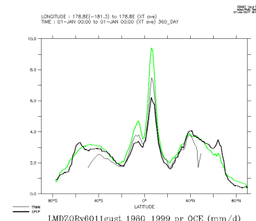
LMDZORv6011gust_1980_1999_oce
