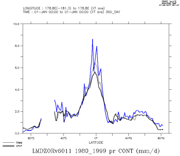
LMDZORv6011_1980_1999_con
