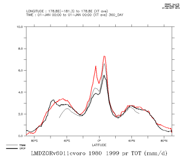
LMDZORv6011cvoro_1980_1999_tot
