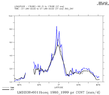
LMDZORv6011bosq.1980_1999_con
