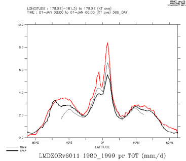
LMDZORv6011_1980_1999_tot
