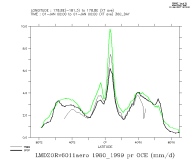
LMDZORv6011aero.1980_1999_oce
