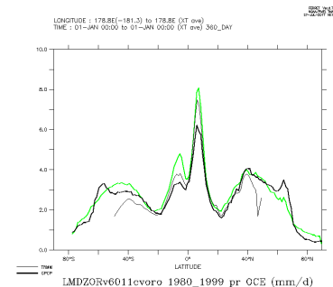
LMDZORv6011cvoro_1980_1999_oce
