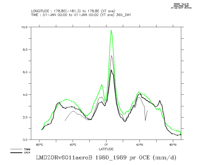
LMDZORv6011aeroB.1980_1989_oce
