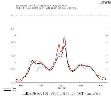
LMDZORv6010J_1980_1999_tot
