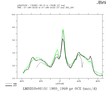
LMDZORv6010J_1980_1999_oce
