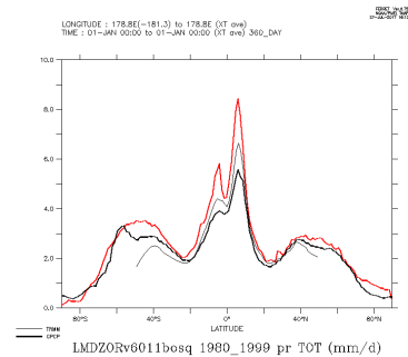
LMDZORv6011bosq.1980_1999_tot
