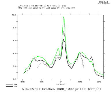
LMDZORv6011OrotkeA.1980_1999_oce
