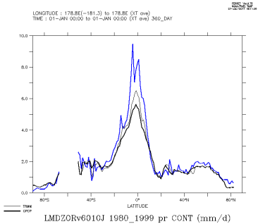
LMDZORv6010J_1980_1999_con
