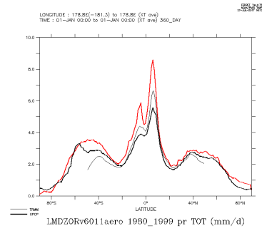
LMDZORv6011aero.1980_1999_tot
