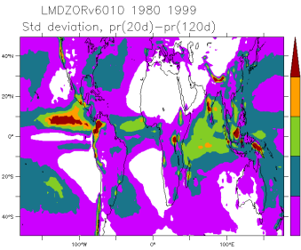
LMDZORv601D_1980_1999_is
