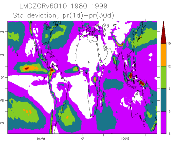
LMDZORv601D_1980_1999_hf
