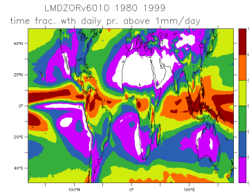
LMDZORv601D_1980_1999_nd
