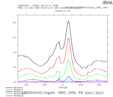
LMDZORv6010epwb_1980_1999_zon
