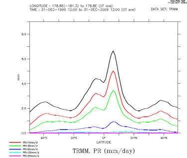
TRMM_zon
