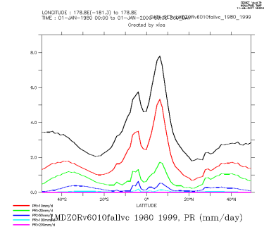
LMDZORv6010fallvc_1980_1999_zon
