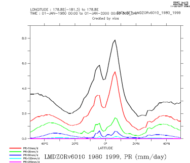
LMDZORv601D_1980_1999_zon
