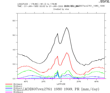
LMDZ607svn2761_1980_1999_zon
