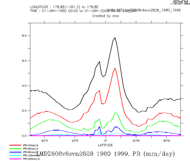
LMDZ608v6svn2828_1980_1999_zon
