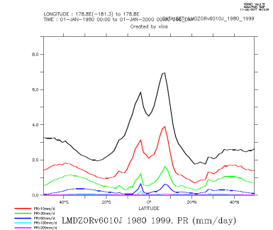
LMDZORv6010J_1980_1999_zon
