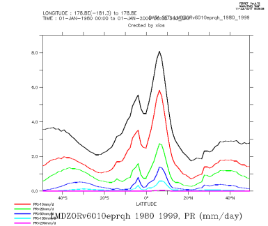
LMDZORv6010eprqh_1980_1999_zon
