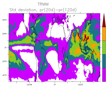
TRMM_is
