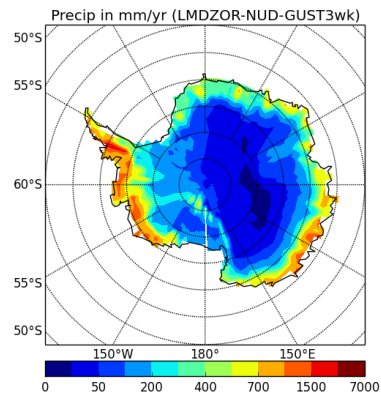
precipSH-LMDZOR-NUD-GUST3wk
