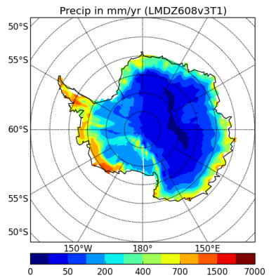
precipSH-LMDZ608v3T1
