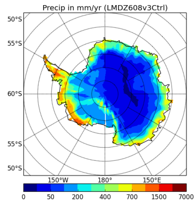
precipSH-LMDZ608v3Ctrl
