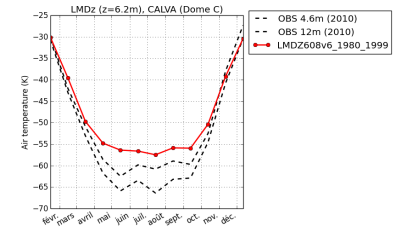
tempDC-LMDZ608v6_1980_1999
