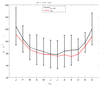
LWdn_DC_LMDZ608v6_1980_1999
