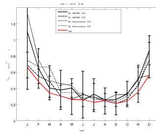
prw_DC_LMDZ608v6_1980_1999
