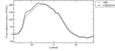
rtczon
