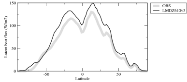
hffszon
