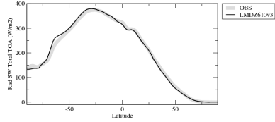
rsttzon
