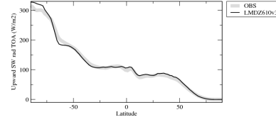
rsutczon
