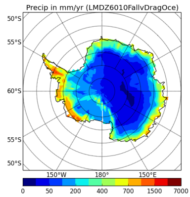
precipSH-LMDZ6010FallvDragOce
