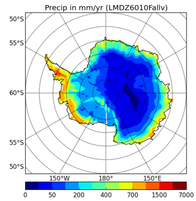
precipSH-LMDZ6010Fallv
