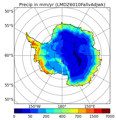
precipSH-LMDZ6010FallvAdjwk
