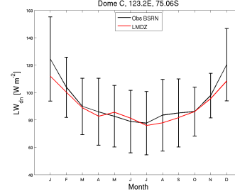
LWdnSFC_DC_CM61-LR-amip-2000_1998_2007
