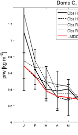
prw_DC_CM6015-LR-amip-split-02_1999_2008
