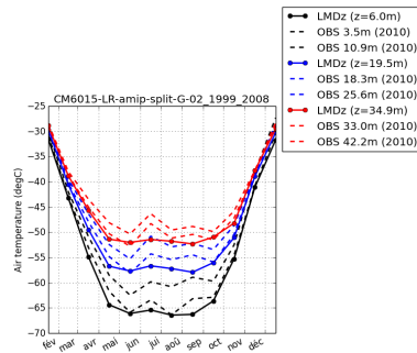
tempDC-CM6015-LR-amip-split-G-02_1999_2008
