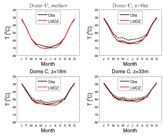
temp_DC_CM6015-LR-amip-split-02_1999_2008
