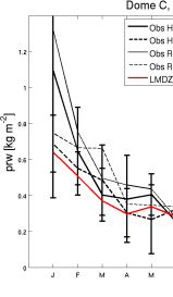
prw_DC_CM61-LR-amip-2000_1998_2007
