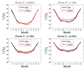
temp_DC_CM61-LR-amip-2000_1998_2007
