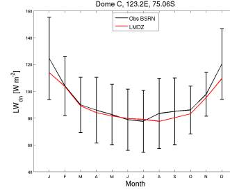
LWdnSFC_DC_CM6015-LR-amip-split-02_1999_2008
