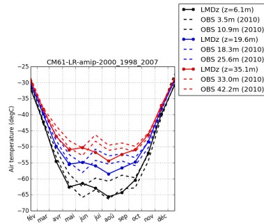
tempDC-CM61-LR-amip-2000_1998_2007
