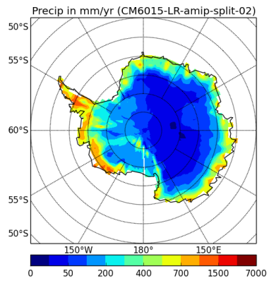
precipSH-CM6015-LR-amip-split-02
