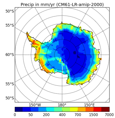
precipSH-CM61-LR-amip-2000
