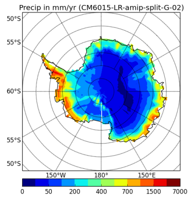
precipSH-CM6015-LR-amip-split-G-02
