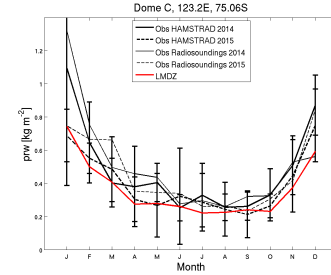
LWdnSFC_DC_CM6011.3-LR-amip-trigB-G-02_1999_2008
