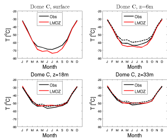
temp_DC_CM6011.3-LR-amip-G-02_1999_2008
