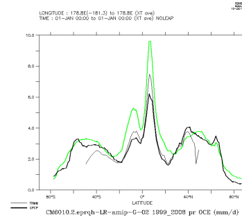
CM6010.2.eprqh-LR-amip-G-02_1999_2008_oce
