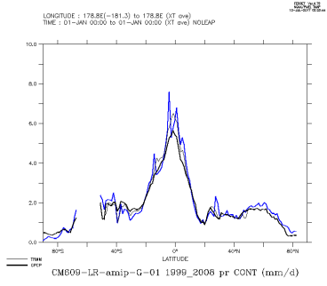
CM609-LR-amp-G-01_1999_2008.con
