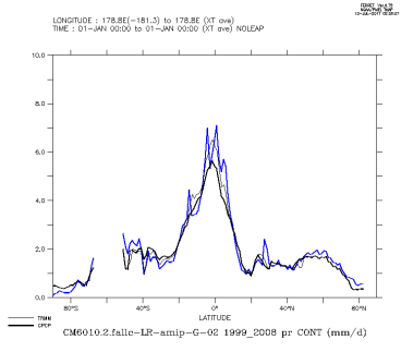
CM6010.2.fallc-LR-amp-G-02_1999_2008.con
