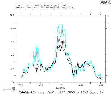
CM609-LR-amp-G-01_1999_2008.mix
