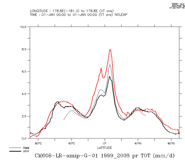
CM608-LR-amp-G-01_1999_2008.tot
