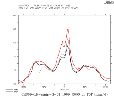
CM609-LR-amp-G-01_1999_2008.tot
