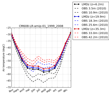
tempDC-CM608-LR-amip-01_1999_2008
