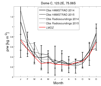
prw_DC_CM609-LR-amip-01_1999_2008
