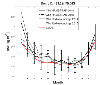
prw_DC_CM608-LR-amip-01_1999_2008
