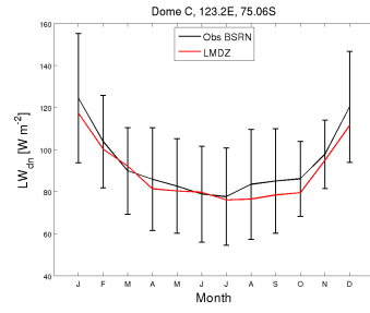
LWdnSFC_DC_CM609-LR-amip-G-01_1999_2008
