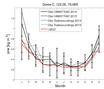
prw_DC_CM608-LR-amip-G-01_1999_2008
