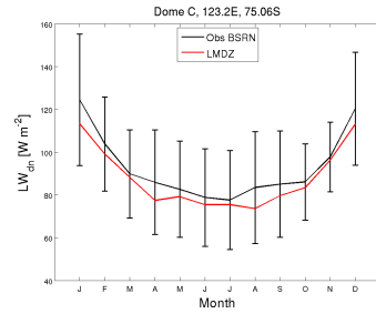
LWdnSFC_DC_CM609-LR-amip-01_1999_2008
