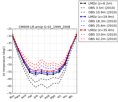
tempDC-CM609-LR-amip-G-01_1999_2008
