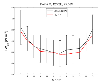
LWdnSFC_DC_CM608-LR-amip-G-01_1999_2008
