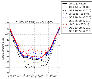
tempDC-CM609-LR-amip-01_1999_2008
