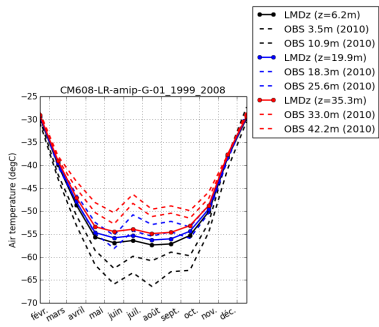
tempDC-CM608-LR-amip-G-01_1999_2008
