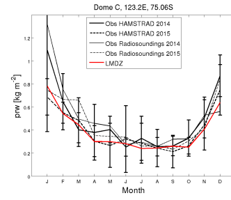
prw_DC_CM609-LR-amip-G-01_1999_2008
