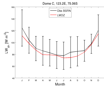
LWdnSFC_DC_CM608-LR-amip-01_1999_2008
