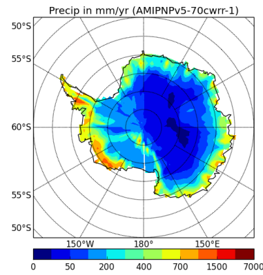
precipSH-AMIPNPv5-70cwrr-1
