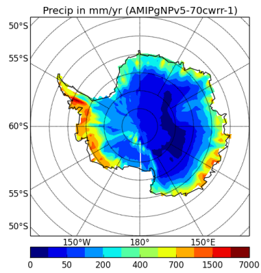
precipSH-AMIPgNPv5-70cwrr-1
