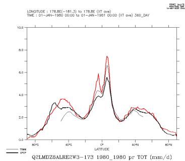
Q2LMDZ6ALRE2W3-173.1980_1980_tot
