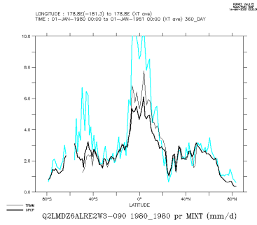
Q2LMDZ6ALRE2W3-090_1980_1980_mix
