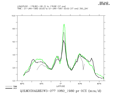
Q2LMDZ6ALRE2W3-077.1980.1980_oce
