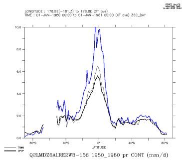
Q2LMDZ6ALRE2W3-156.1980_1980_con
