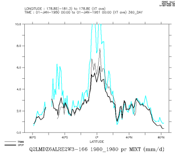
Q2LMDZ6ALRE2W3-166.1980.1980_mix
