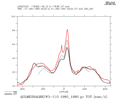
Q2LMDZ6ALRE2W3-210.1980.1980_tot
