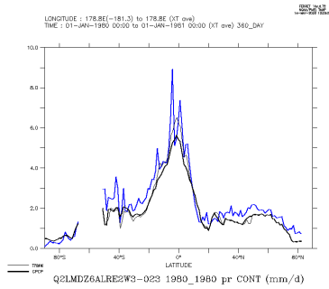
Q2LMDZ6ALRE2W3-023.1980.1980_con
