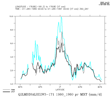
Q2LMDZ6ALRE2W3-171_1980_1980_mix
