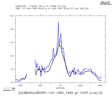
Q2LMDZ6ALRE2W3-210.1980.1980_con
