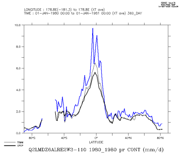
Q2LMDZ6ALRE2W3-110.1980.1980_con
