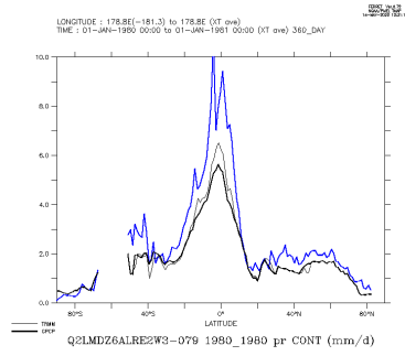
Q2LMDZ6ALRE2W3-079.1980.1980_con
