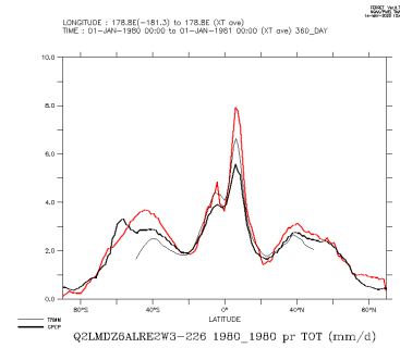
Q2LMDZ6ALRE2W3-226.1980.1980_tot
