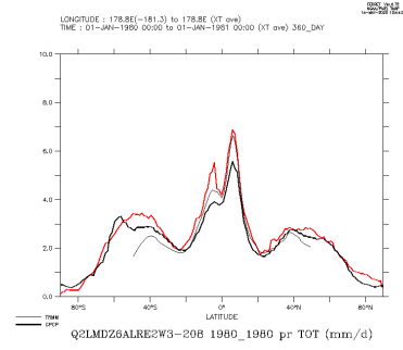
Q2LMDZ6ALRE2W3-208.1980.1980_tot
