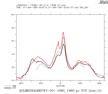
Q2LMDZ6ALRE2W3-001_1980_1980_tot
