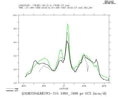
Q2LMDZ6ALRE2W3-224.1980.1980_oce
