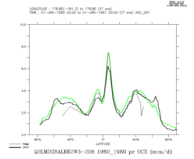
Q2LMDZ6ALRE2W3-208.1980.1980_oce
