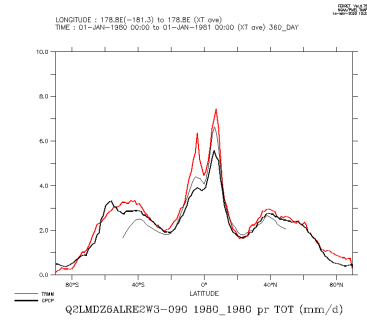
Q2LMDZ6ALRE2W3-090_1980_1980_tot
