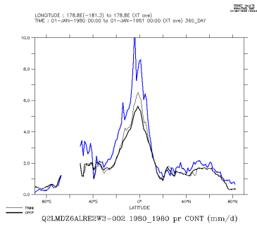
Q2LMDZ6ALRE2W3-002_1980_1980_con
