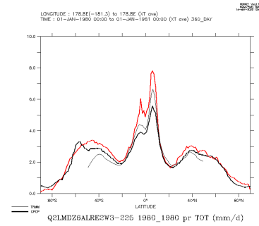
Q2LMDZ6ALRE2W3-225.1980.1980_tot
