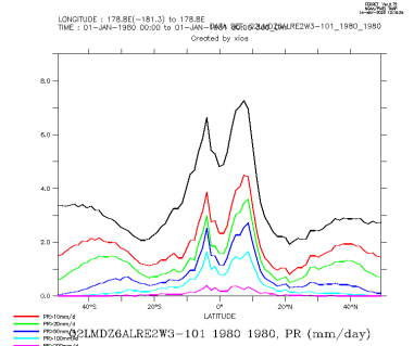
Q2LMDZ6ALRE2W3-101_1980_1980_zon
