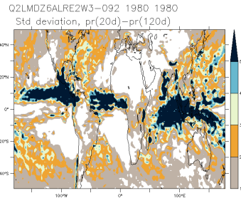
Q2LMDZ6ALRE2W3-092_1980_1980_is
