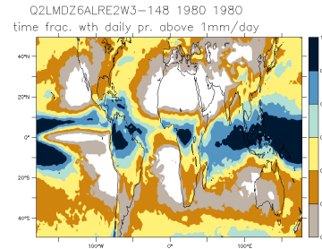
Q2LMDZ6ALRE2W3-148_1980_1980_nd
