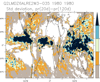
Q2LMDZ6ALRE2W3-035_1980_1980_is
