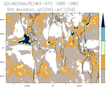
Q2LMDZ6ALRE2W3-072_1980_1980_is
