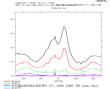
Q2LMDZ6ALRE2W3-171_1980_1980_zon
