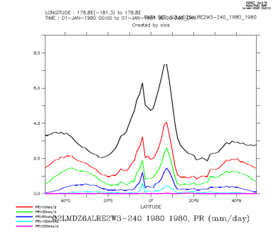
Q2LMDZ6ALRE2W3-240_1980_1980_zon
