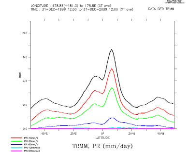
TRMM_zon
