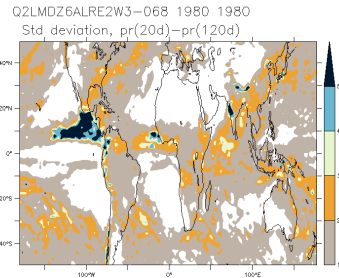
Q2LMDZ6ALRE2W3-068_1980_1980_is
