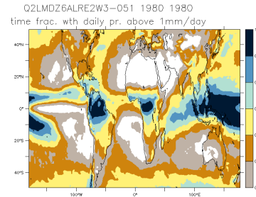
Q2LMDZ6ALRE2W3-051_1980_1980_nd
