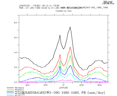
Q2LMDZ6ALRE2W3-090_1980_1980_zon
