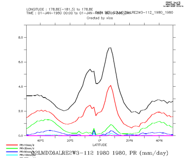
Q2LMDZ6ALRE2W3-112_1980_1980_zon
