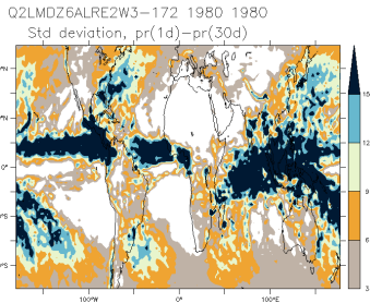
Q2LMDZ6ALRE2W3-172_1980_1980_hf
