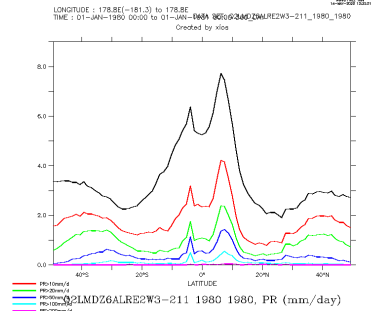
Q2LMDZ6ALRE2W3-211_1980_1980_zon
