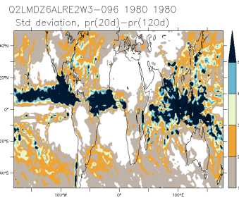
Q2LMDZ6ALRE2W3-096_1980_1980_is
