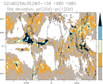
Q2LMDZ6ALRE2W3-136_1980_1980_is
