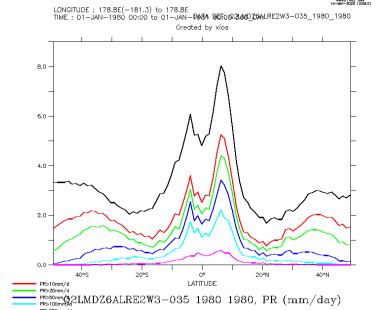
Q2LMDZ6ALRE2W3-035_1980_1980_zon
