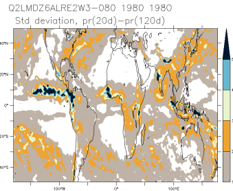
Q2LMDZ6ALRE2W3-080_1980_1980_is
