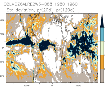
Q2LMDZ6ALRE2W3-088_1980_1980_is
