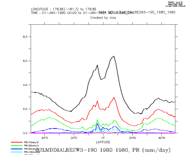
Q2LMDZ6ALRE2W3-190_1980_1980_zon
