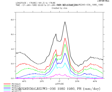
Q2LMDZ6ALRE2W3-036_1980_1980_zon
