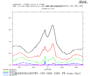
Q2LMDZ6ALRE2W3-158_1980_1980_zon
