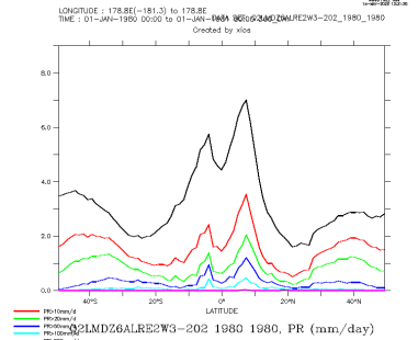
Q2LMDZ6ALRE2W3-202_1980_1980_zon
