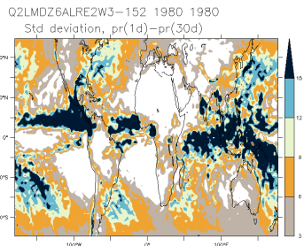
Q2LMDZ6ALRE2W3-152_1980_1980_hf
