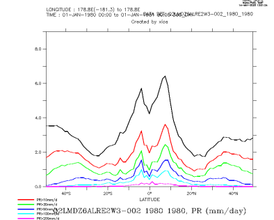
Q2LMDZ6ALRE2W3-002_1980_1980_zon
