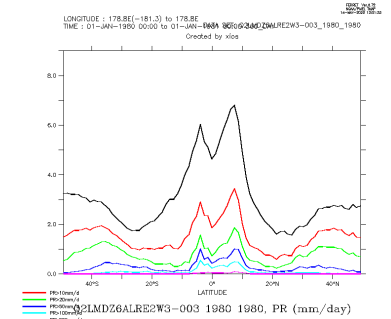
Q2LMDZ6ALRE2W3-003_1980_1980_zon
