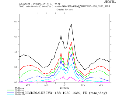
Q2LMDZ6ALRE2W3-188_1980_1980_zon
