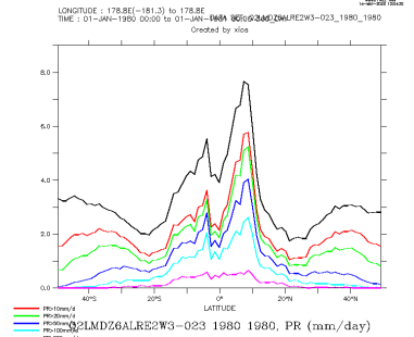
Q2LMDZ6ALRE2W3-023_1980_1980_zon
