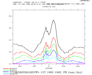
Q2LMDZ6ALRE2W3-137_1980_1980_zon
