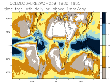
Q2LMDZ6ALRE2W3-239_1980_1980_nd
