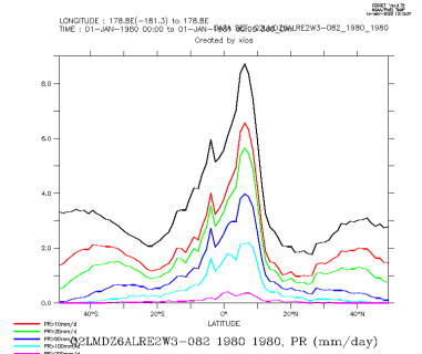
Q2LMDZ6ALRE2W3-082_1980_1980_zon
