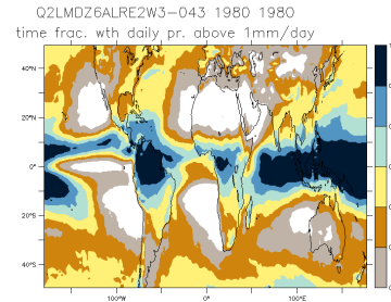
Q2LMDZ6ALRE2W3-043_1980_1980_nd
