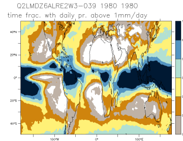
Q2LMDZ6ALRE2W3-039_1980_1980_nd
