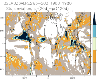
Q2LMDZ6ALRE2W3-202_1980_1980_is
