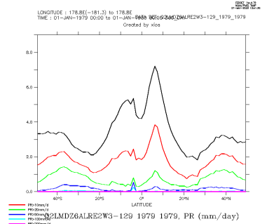
Q2LMDZ6ALRE2W3-129_1979_1979_zon
