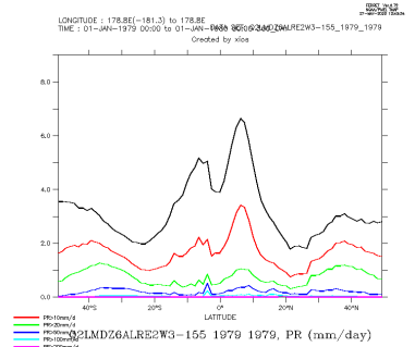
Q2LMDZ6ALRE2W3-155_1979_1979_zon
