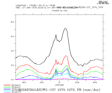
Q2LMDZ6ALRE2W3-237_1979_1979_zon
