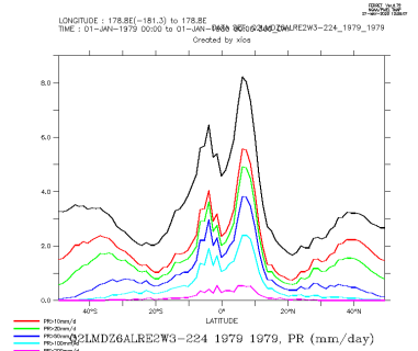
Q2LMDZ6ALRE2W3-224_1979_1979_zon
