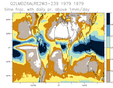
Q2LMDZ6ALRE2W3-239_1979_1979_nd
