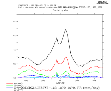
Q2LMDZ6ALRE2W3-163_1979_1979_zon
