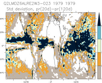
Q2LMDZ6ALRE2W3-023_1979_1979_is
