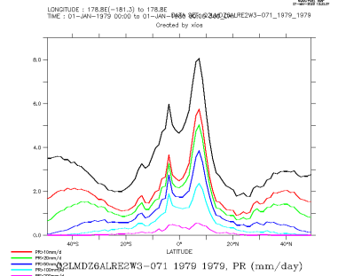
Q2LMDZ6ALRE2W3-071_1979_1979_zon
