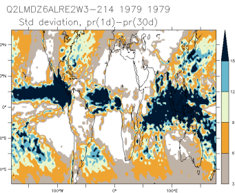
Q2LMDZ6ALRE2W3-214_1979_1979_hf
