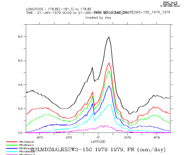
Q2LMDZ6ALRE2W3-150_1979_1979_zon
