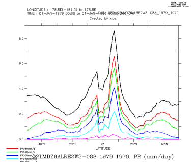
Q2LMDZ6ALRE2W3-088_1979_1979_zon
