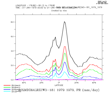
Q2LMDZ6ALRE2W3-181_1979_1979_zon
