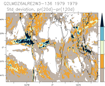
Q2LMDZ6ALRE2W3-136_1979_1979_is
