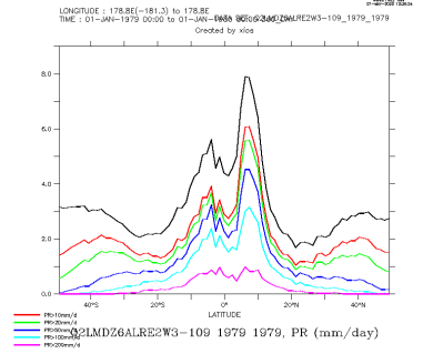
Q2LMDZ6ALRE2W3-109_1979_1979_zon
