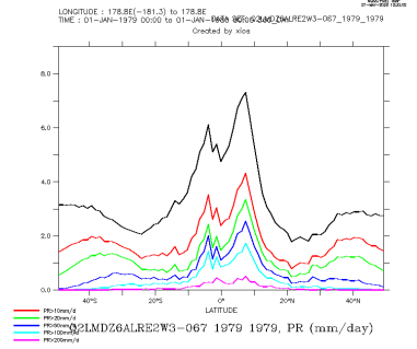
Q2LMDZ6ALRE2W3-067_1979_1979_zon
