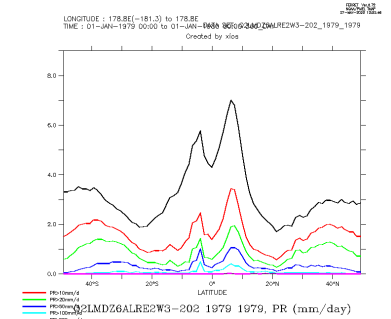
Q2LMDZ6ALRE2W3-202_1979_1979_zon
