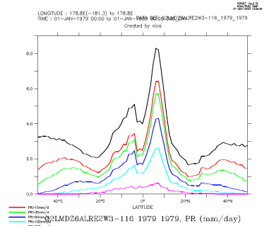
Q2LMDZ6ALRE2W3-116_1979_1979_zon
