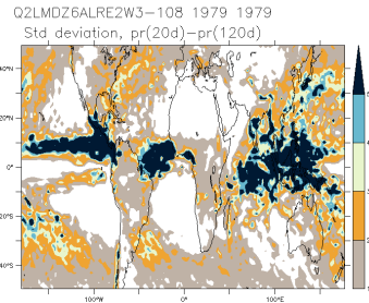
Q2LMDZ6ALRE2W3-108_1979_1979_is
