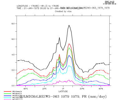
Q2LMDZ6ALRE2W3-063_1979_1979_zon
