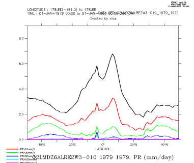
Q2LMDZ6ALRE2W3-010_1979_1979_zon
