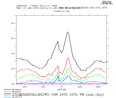
Q2LMDZ6ALRE2W3-208_1979_1979_zon
