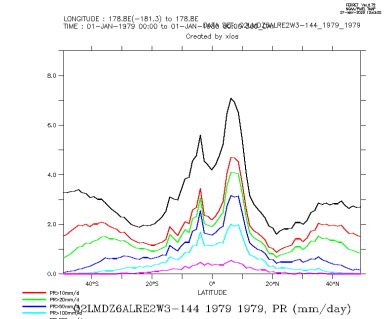
Q2LMDZ6ALRE2W3-144_1979_1979_zon
