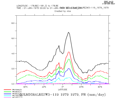
Q2LMDZ6ALRE2W3-119_1979_1979_zon
