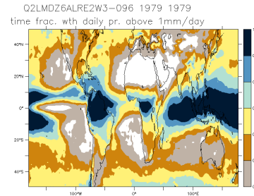
Q2LMDZ6ALRE2W3-096_1979_1979_nd
