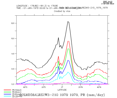
Q2LMDZ6ALRE2W3-210_1979_1979_zon
