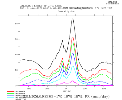
Q2LMDZ6ALRE2W3-170_1979_1979_zon
