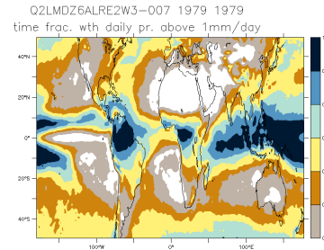
Q2LMDZ6ALRE2W3-007_1979_1979_nd
