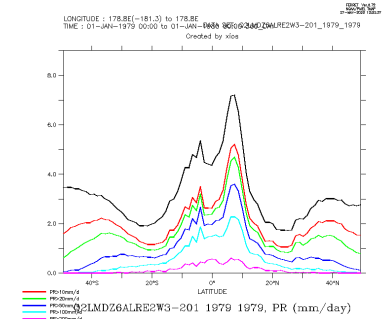
Q2LMDZ6ALRE2W3-201_1979_1979_zon
