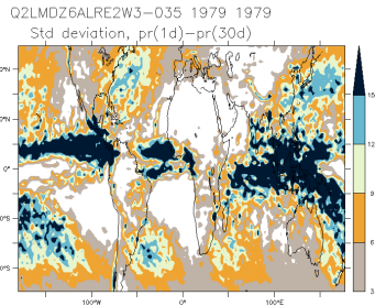
Q2LMDZ6ALRE2W3-035_1979_1979_hf
