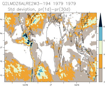
Q2LMDZ6ALRE2W3-194_1979_1979_hf
