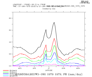
Q2LMDZ6ALRE2W3-090_1979_1979_zon
