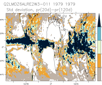
Q2LMDZ6ALRE2W3-011_1979_1979_is
