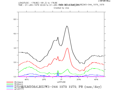
Q2LMDZ6ALRE2W3-044_1979_1979_zon
