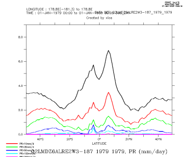
Q2LMDZ6ALRE2W3-187_1979_1979_zon
