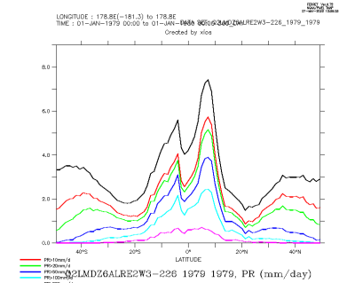
Q2LMDZ6ALRE2W3-226_1979_1979_zon
