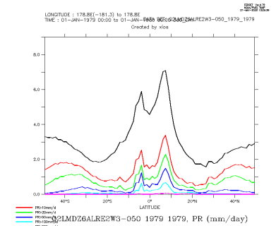
Q2LMDZ6ALRE2W3-050_1979_1979_zon
