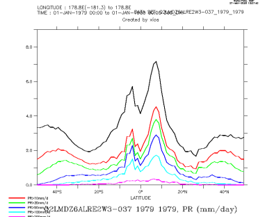
Q2LMDZ6ALRE2W3-037_1979_1979_zon
