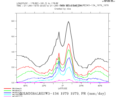
Q2LMDZ6ALRE2W3-134_1979_1979_zon
