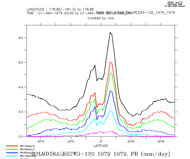
Q2LMDZ6ALRE2W3-120_1979_1979_zon
