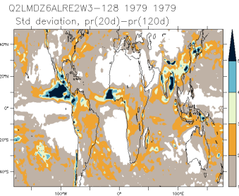
Q2LMDZ6ALRE2W3-128_1979_1979_is
