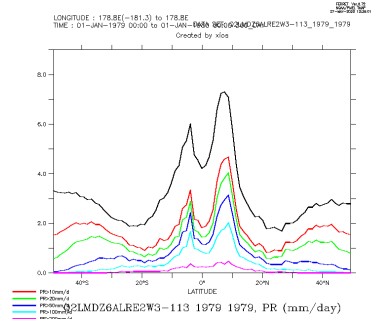
Q2LMDZ6ALRE2W3-113_1979_1979_zon
