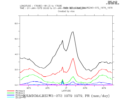
Q2LMDZ6ALRE2W3-072_1979_1979_zon
