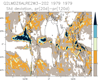
Q2LMDZ6ALRE2W3-202_1979_1979_is
