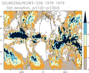
Q2LMDZ6ALRE2W3-039_1979_1979_hf
