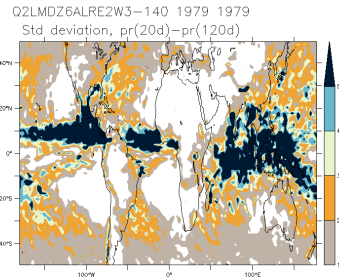
Q2LMDZ6ALRE2W3-140_1979_1979_is
