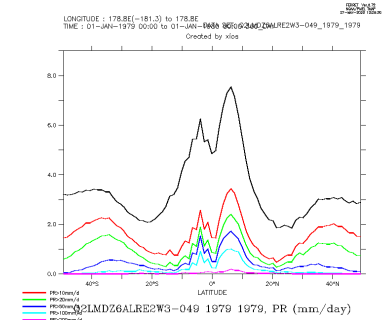
Q2LMDZ6ALRE2W3-049_1979_1979_zon
