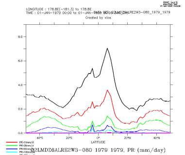
Q2LMDZ6ALRE2W3-080_1979_1979_zon
