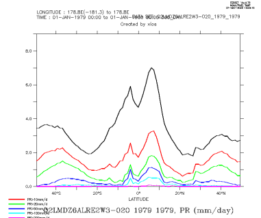
Q2LMDZ6ALRE2W3-020_1979_1979_zon
