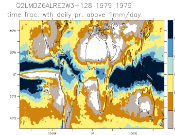
Q2LMDZ6ALRE2W3-128_1979_1979_nd
