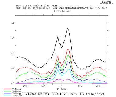
Q2LMDZ6ALRE2W3-222_1979_1979_zon
