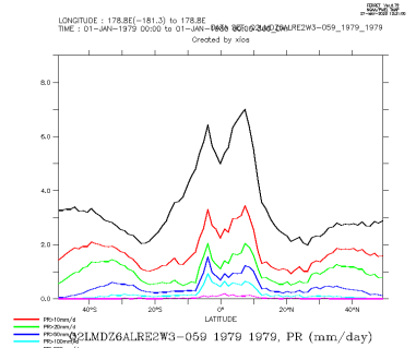
Q2LMDZ6ALRE2W3-059_1979_1979_zon
