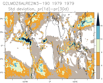
Q2LMDZ6ALRE2W3-190_1979_1979_hf
