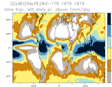
Q2LMDZ6ALRE2W3-176_1979_1979_nd
