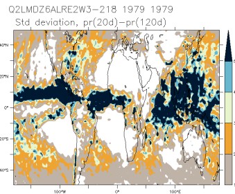
Q2LMDZ6ALRE2W3-218_1979_1979_is
