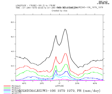
Q2LMDZ6ALRE2W3-106_1979_1979_zon
