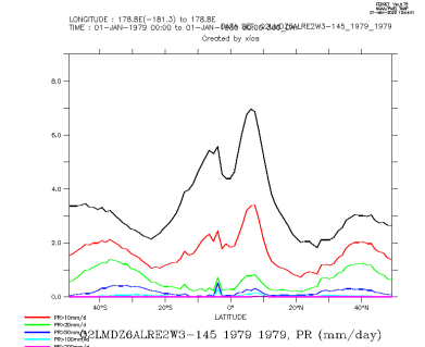
Q2LMDZ6ALRE2W3-145_1979_1979_zon
