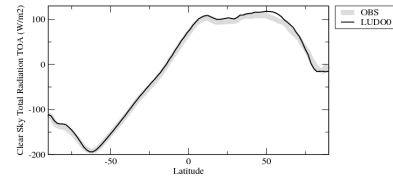
rttcszon
