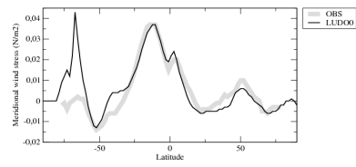
tauvzon
