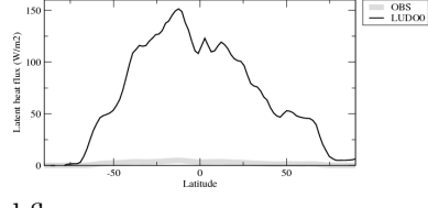
hflszon
