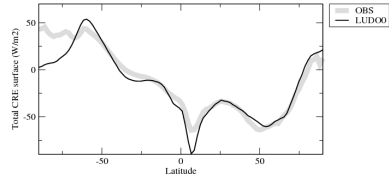
cretlcalipszon
