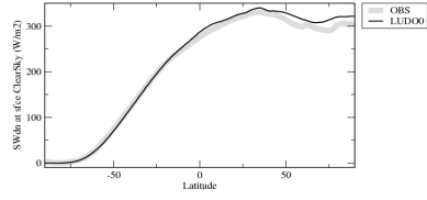
rsdscszon
