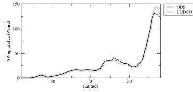
rsuszon
