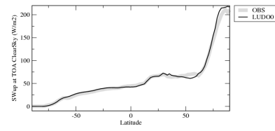
rsutcszon
