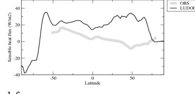
hflsszon
