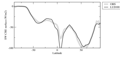
crelcalipszon
