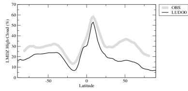
chlzon
