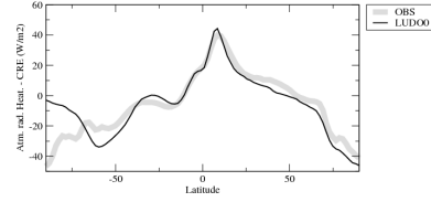
rahcrezon
