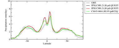
przn
