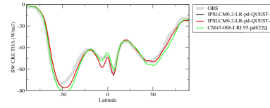
crestzn
