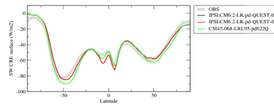
crosszon
