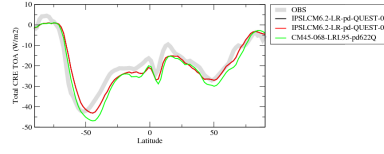
crettzn
