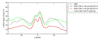
chlhzon
