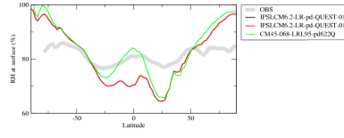
hurszon
