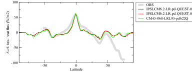
hfnsszon
