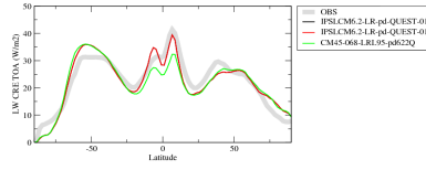
creltzon
