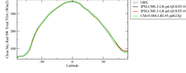
rsttcrezon
