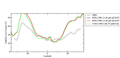
cllzn
