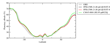
albtzon
