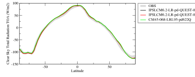
rttcszon
