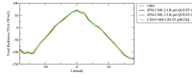
rttzn
