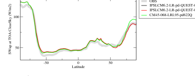
rsutcscrezon
