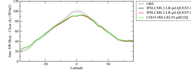
rsahcscrezon
