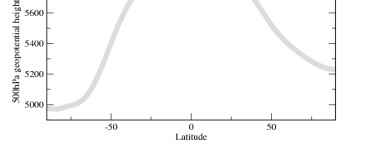
zg500zon
