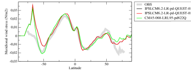
tauvzon
