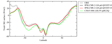
cretzon
