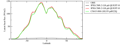
hfllszon
