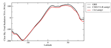
rttcszon
