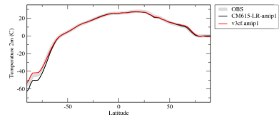
taszon
