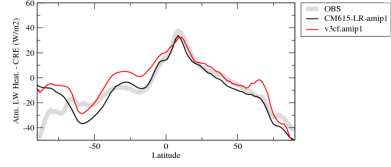
rlahcrezon
