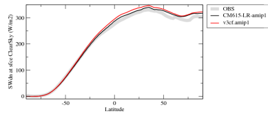
rsdscszone
