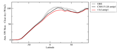
rsahcszone
