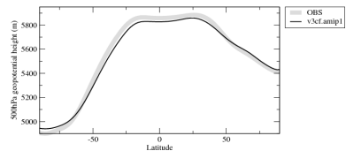
zg500zon
