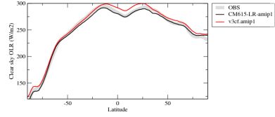
rlutcszone
