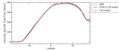
rsttcszone
