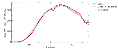
rsttzone
