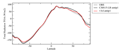
rttzon
