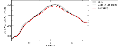
rldscszone
