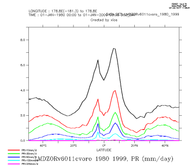
LMDZORv6011cvoro_1980_1999_zon
