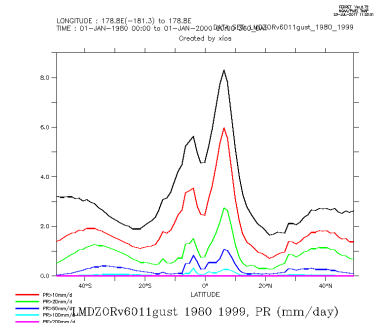
LMDZORv6011gust_1980_1999_zon
