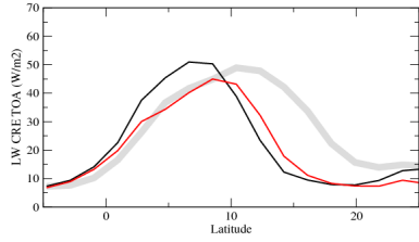
cretlzon
