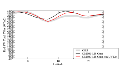
rsttzn
