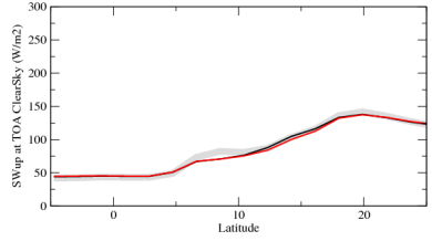
rsutcszn
