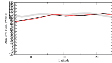
rsahczon
