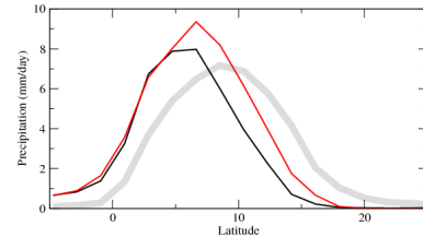
przon
