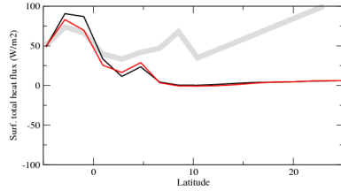
hfnszon
