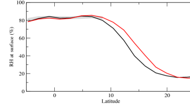
hurszon
