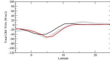
crettzn
