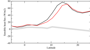
hfsszon
