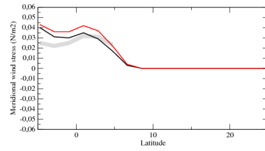
tauvzn
