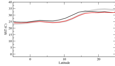
sstzn
