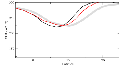
rlutczon
