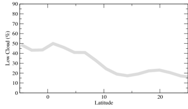
cllcalipsozon
