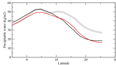
prwzon
