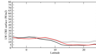
crelszon
