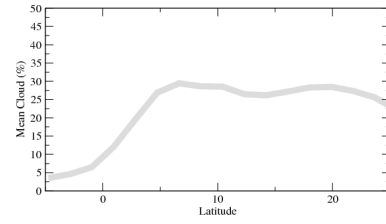
clmcalipsozon
