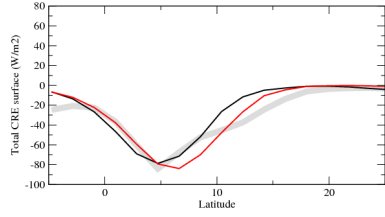
cretszon
