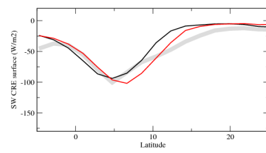
cresszon
