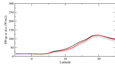
rsuszn
