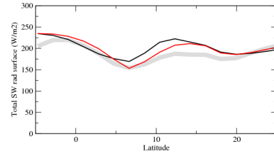
rstczon
