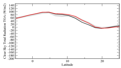
rttcszn
