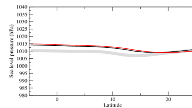
pslzon
