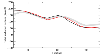
rtszn
