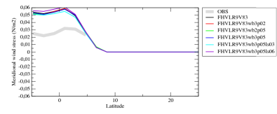
tauvzon
