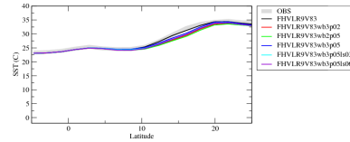
rstzon
