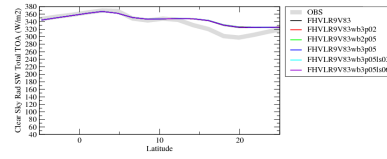
rdszczon
