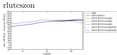
rlutcszon
