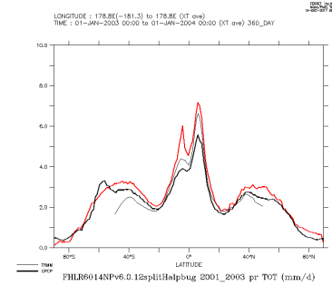
FHLR6014NPv6.0.12splitHalpbug_2001_2003_tot
