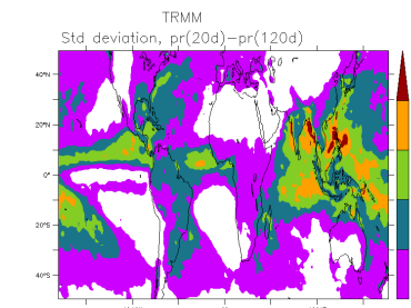
TRMM_is
