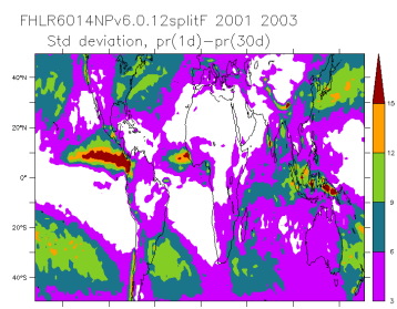
FHLR6014NPv6.0.12split_2001_2003_hf
