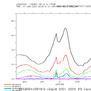
FHLR6014NPv6.0.12split_2001_2003_zon
