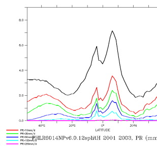
FHLR6014NPv6.0.12splitH
