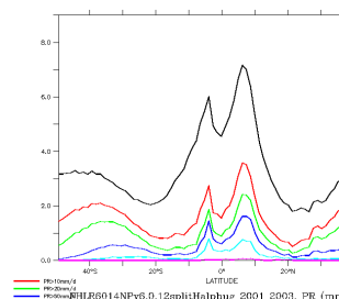
FHLR6014NPv6.0.12splitHalpbug
