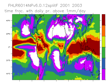
FHLR6014NPv6.0.12split_2001_2003_nd
