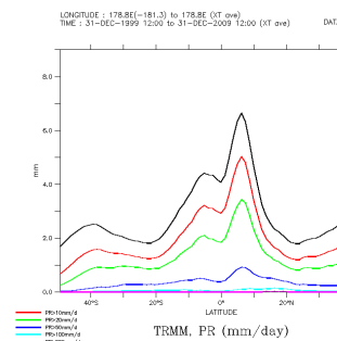
TRMM_zon
