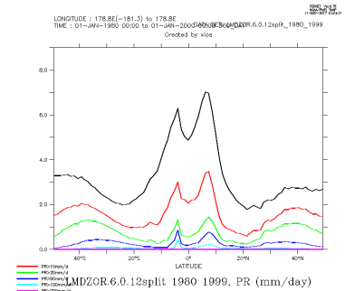
LMDZOR.6.0.12split_1980_1999_zon
