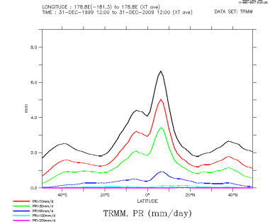
TRMM_zon
