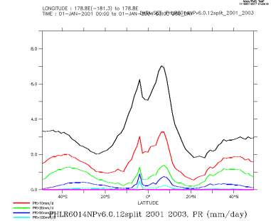
FHLR6014NPv6.0.12split_2001_2003_zon
