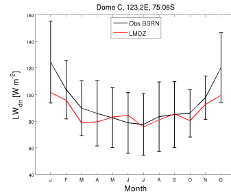
LWdnSFC_DC_FHLR9V60102conmy_2000_2000
