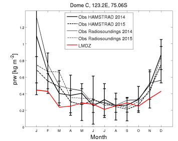
prw_DC_FHLR9V60102conmy_2000_2000
