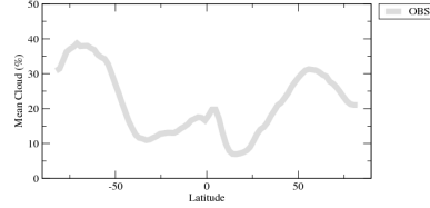
clmcalipsozn
