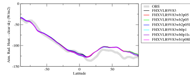
rahcszozn
