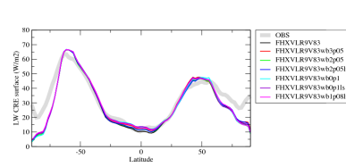
crelszozn
