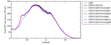
rsdszone
