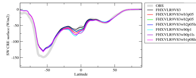
crosszozn
