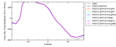
rsutcrezon
