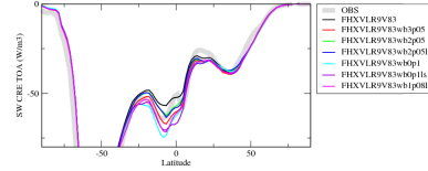
crestzozn
