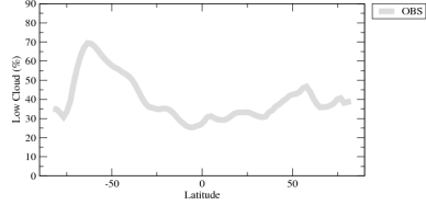
cllcalipsozn
