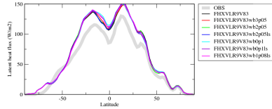
hflszozn
