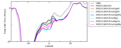
crettzozn
