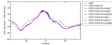
rahcrezozn
