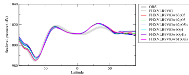
pslzozn
