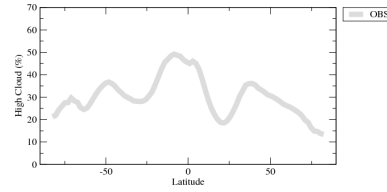
clhcalipsozn
