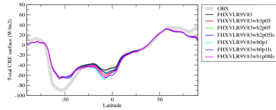
cretszozn
