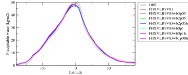
prwzozn
