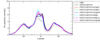
przozn
