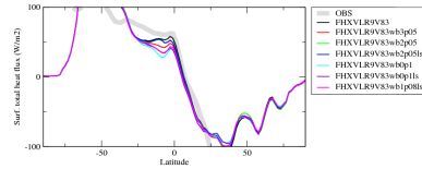
hfnszozn
