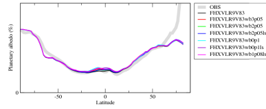
albtzozn
