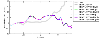
hfnstzozn
