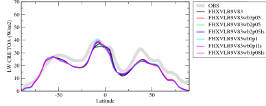
cretzozn
