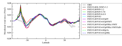
tauvzon
