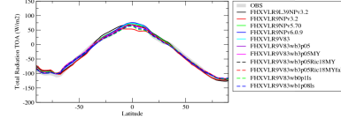
rttsczon
