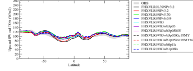
rsutzon
