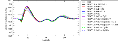
tauozon
