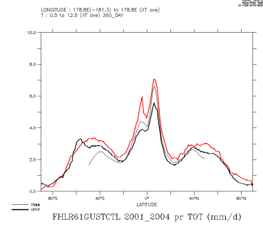
FHLR61GUSTCTL_2001_2004_tot
