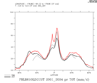
FHLR61OLDGUST_2001_2004_tot
