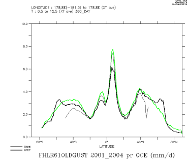
FHLR61OLDGUST_2001_2004_oce
