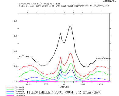
FHLR61MILLER_2001_2004_zon
