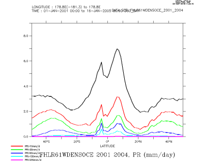
FHLR61WDENSOCE_2001_2004_zon
