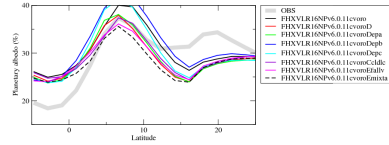
albtzn
