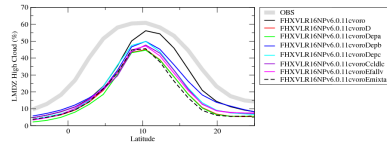
clhzon
