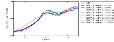
rlahczon
