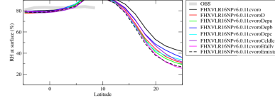
hurszon
