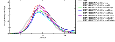
przn
