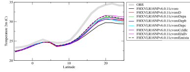
taszon
