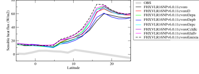
hfsszon
