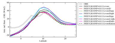
rahcrezon
