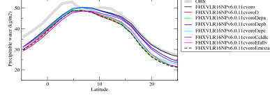
prwzon
