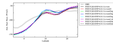
rahczon
