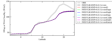
rsutcszon
