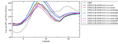
rsutczon
