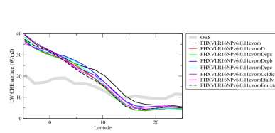
crelson
