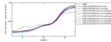
rahcszon
