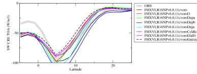
crestzn
