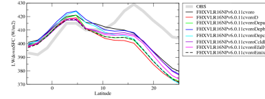
rldsczon
