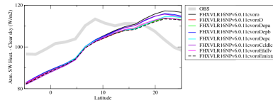
rsahcszon
