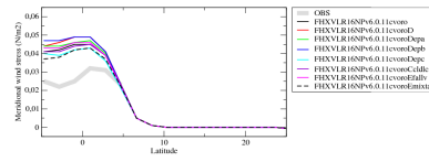
tauvzon
