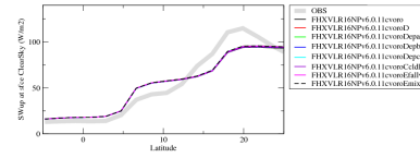
rsttzn
