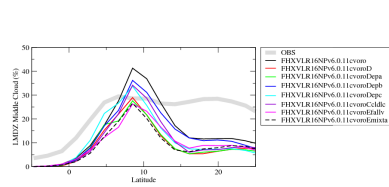
clmzn
