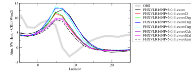
rsahczon
