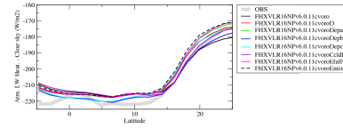
rlahcszon
