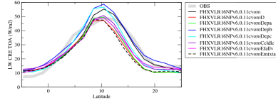
cretzon
