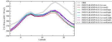
rldscszon
