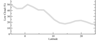
clcalipsozon
