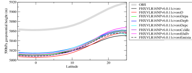
zg500zon
