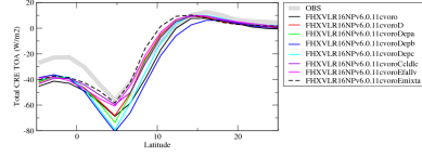
crettzn
