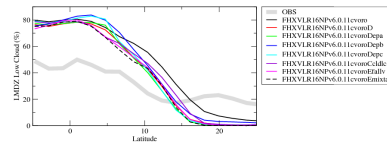
cllzn
