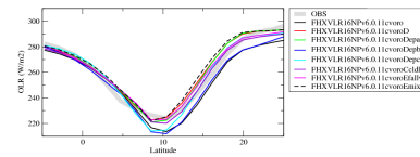
rlutczon
