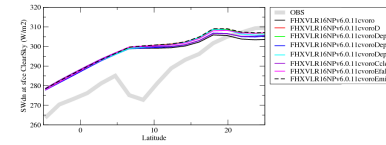
rsdszon
