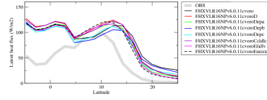
hfhszon
