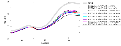
sstzon
