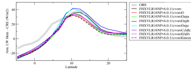
rlahcrezon
