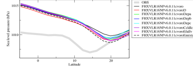
pslzn
