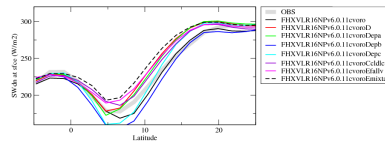
rsdszon
