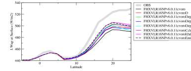
rluszon
