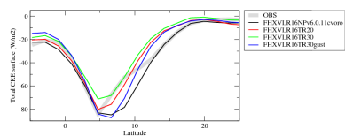
ctotalcalipsozon
