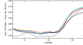
ralhcszon
