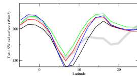
rsttazon
