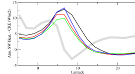
rsahcrezon
