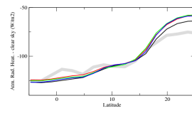
rahcszon
