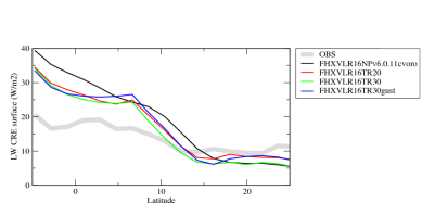
crelcalipsozon
