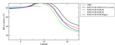
rhcalipsozon
