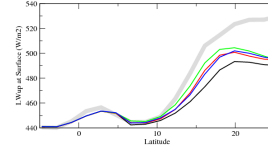
rluszon
