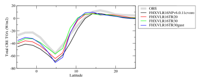
ctotalzon
