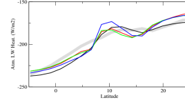
ralhazon
