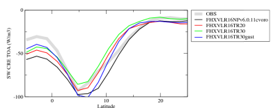
cswzon
