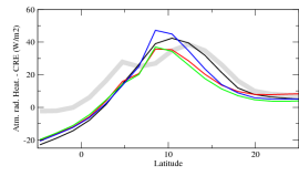
rahcrezon
