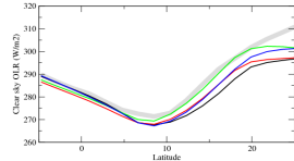
rlutcszon
