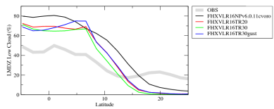
clzon
