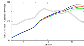
rsahcszon
