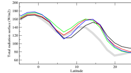
rtszon
