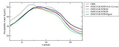
prwcalipsozon
