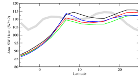
rsahazon
