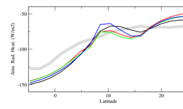
rahazon
