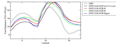
rttazon
