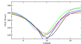
rlutazon
