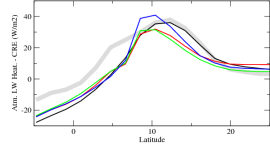
ralhcrezon
