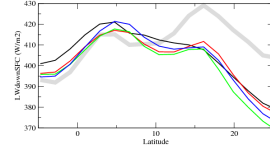
rldscszon
