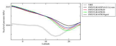
pslcalipsozon
