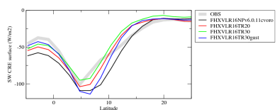
cswcalipsozon
