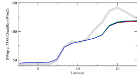
rsutcszon
