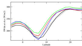
rsdszon
