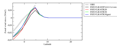
tauazon
