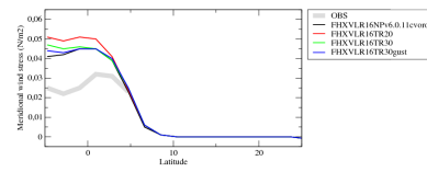
tauvazon
