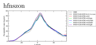
prwzon
