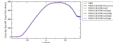
rsttazon
