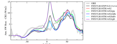
rsahcrezon
