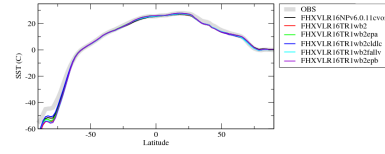
sstzn
