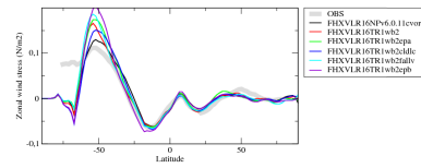
tauzzn
