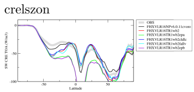
crelazon
