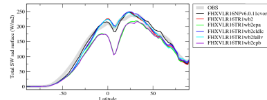
rstscszon
