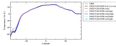
taszn
