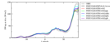
rsutczon
