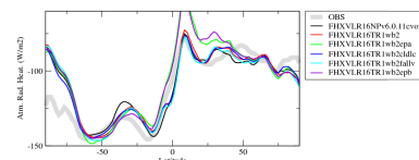
rahczon
