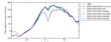
rtszon
