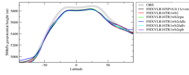
zg500zn
