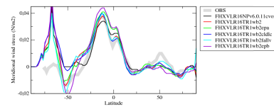
tauvzn
