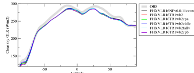
rlutscszon
