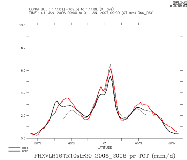
FHXVLR16TR10str20_2006_2006_tot
