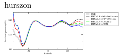
pslzon
