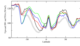
rsutzon
