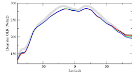
rlutcszon
