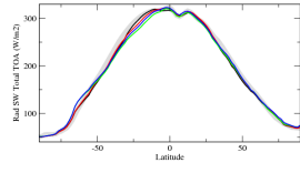
rsttzon
