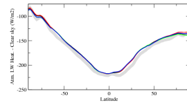
ralahcszon
