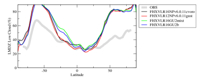
chlcalipszon
