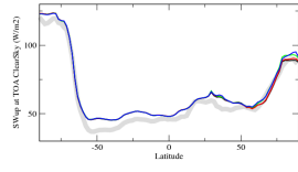
rsutcszon
