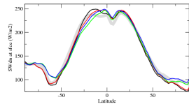
rsdszon
