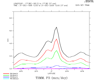
TRMM_zon
