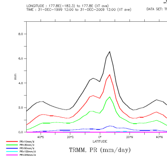
TRMM_zon
