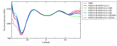
psl3zon
