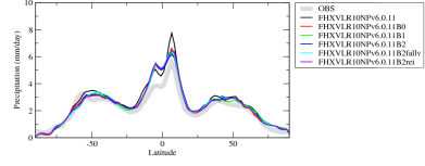
pr3zon
