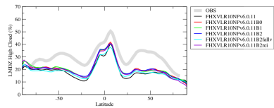
clh3zon
