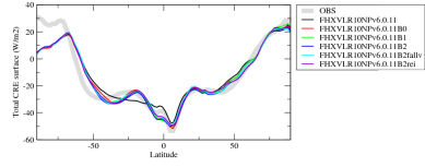
cret3zon
