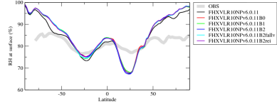
hurs3zon
