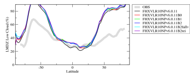
cll3zon
