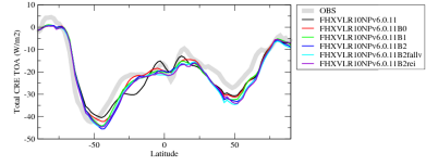
cret3zon
