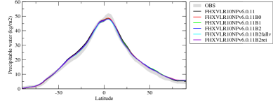
prw3zon
