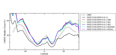
clm3zon
