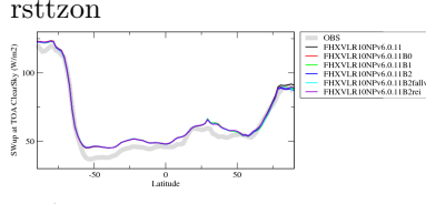
rsutscszon
