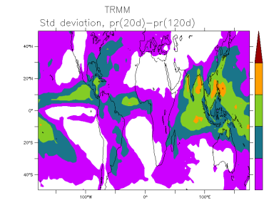
TRMM_is
