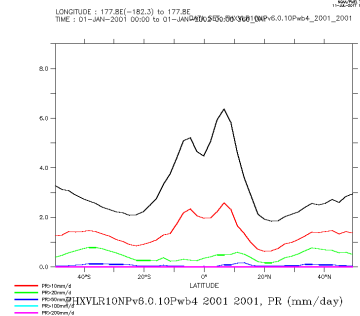
FHXVLR10NPv6.0.10Pwb4_2001_2001_zon
