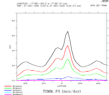
TRMM_zon
