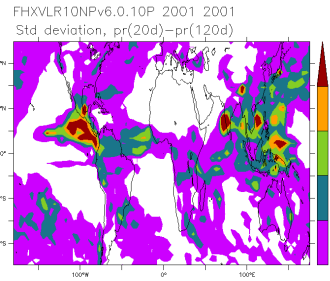
TRMM_is
