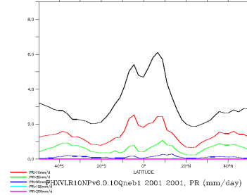
FHXVLR10NPv6.0.10Qneb1_2001_2001_nd
